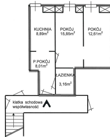
UPROSZCZONY SZKIC LOKALU MIESZKALNEGO NR 9 BOLESŁAWIEC ul. Rynek 29/30 piętrem 2 piętra działka nr 271, IX obręb ewidencyjny instalacje: elektryczna, wodna, kanalizacyjna, gazowa wysokość pomieszczeń - powyżej 2,50m; powierzchnia użytkowa - 48,52m 2
