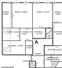
UPROSZCZONY SZKIC LOKALU MIESZKALNEGO NR 10 BOLESŁAWIEC ul. Warszawska 1 poziom 2 piętra
